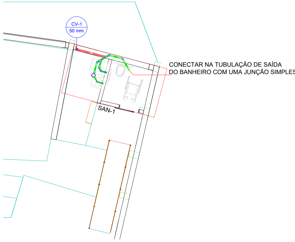
PLANTA BAIXA - LAVANDERIA ESC. 1:100
