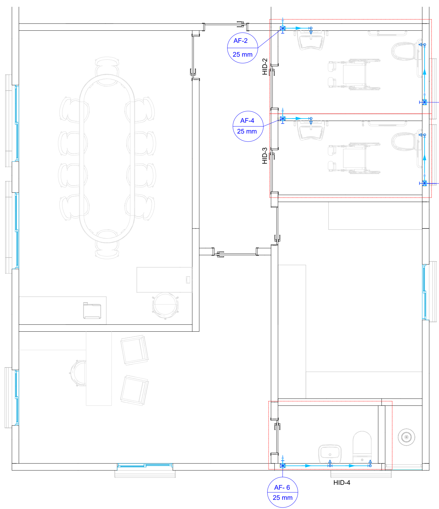
PLANTA BAIXA - HIDRÁULICO TÉRREO ADM ESC. 1:50
