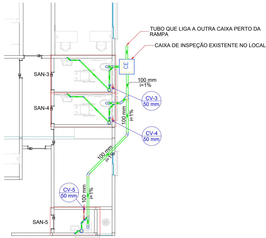
PLANTA BAIXA - TÉRREO ADM ESC. 1:100
