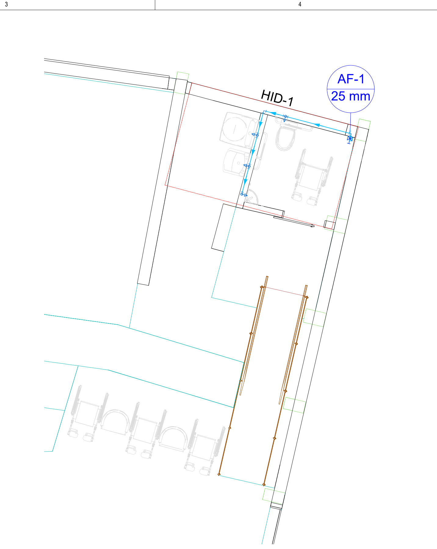
PLANTA BAIXA - HIDRÁULICO ÁREA DE SERVIÇO E SANITÁRIO PCD ESC. 1:50
