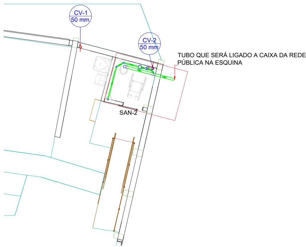
PLANTA BAIXA - SANITÁRIO ESC. 1:100
