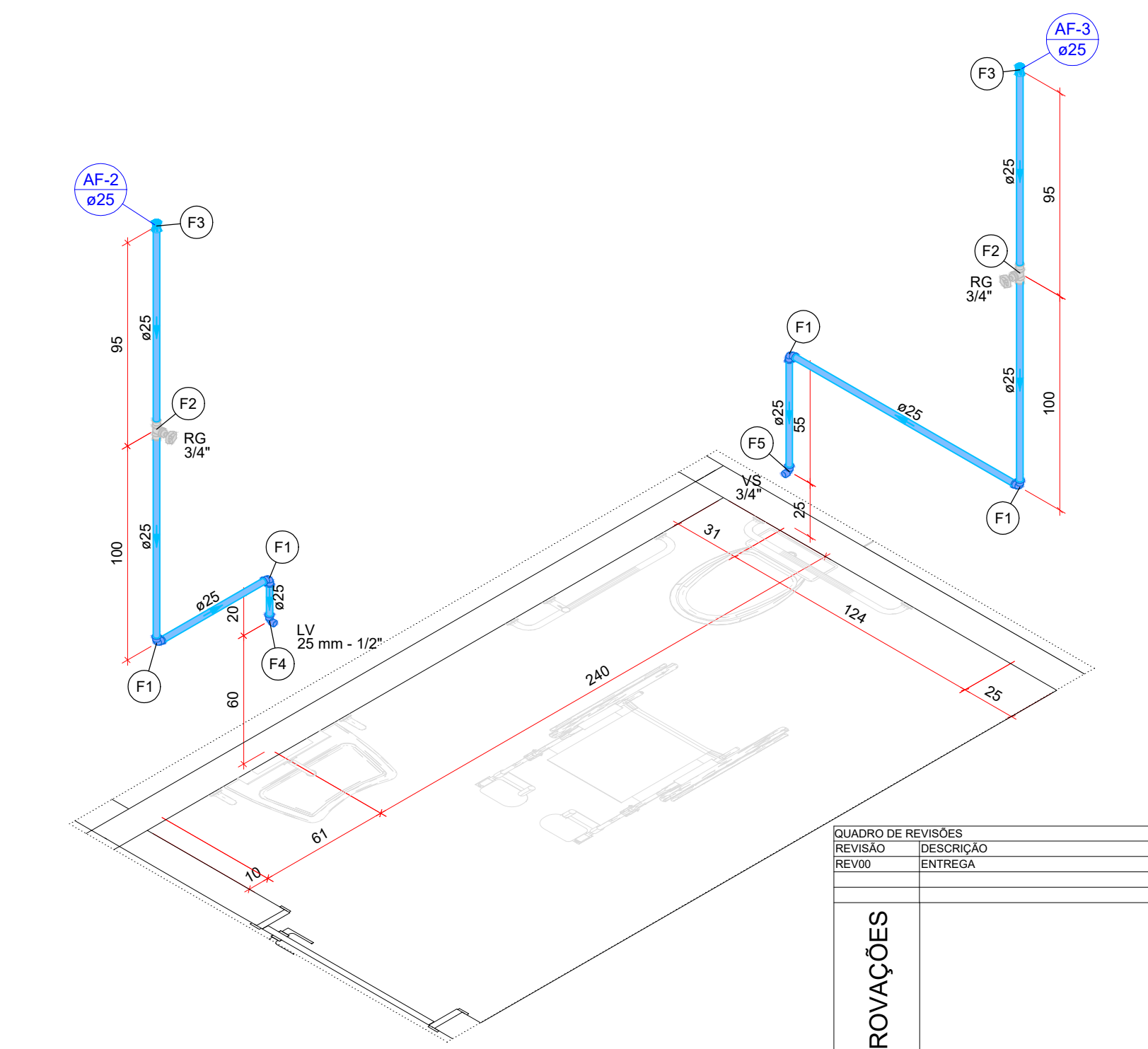
DETALHE HID 2 ESC. 1:25
